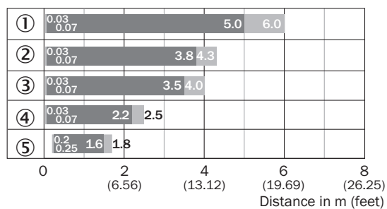
触发感应距离图表 GL6, GL6G
